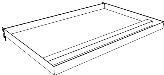
P01A – Zastrešenie š.1000 × hl.650 × v.55 mm, vrátane žiarivkového telesa OPPL FIB 873, 21 W modul 1000 Cena bez DPH: 75,60 €
