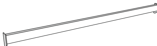
P08 – Traverza na držiaky krovinorezov a reťazových píl 1000 × 60 × 110mm
