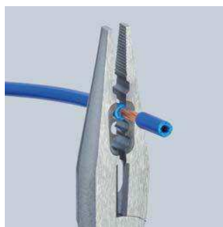
Abisolieren
