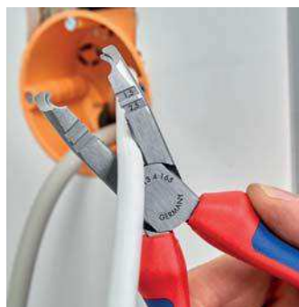
Schneiden von Kabeln bis Ø 13 mm
