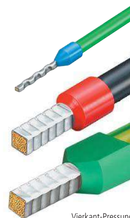
Vierkant-Pressung
