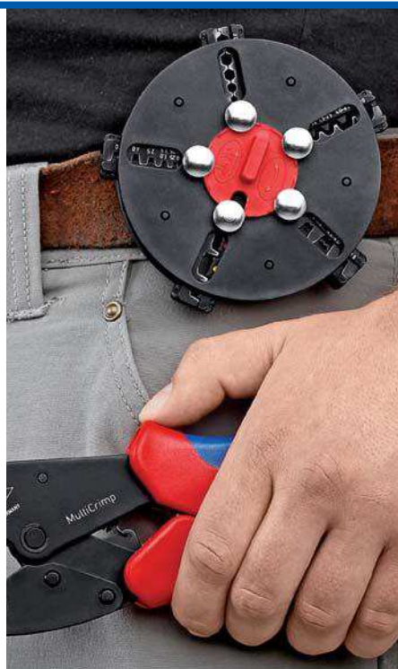
Magazin für Crimpeinsätze kann am Gürtel getragen werden
