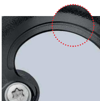
Präzisionsgefräste und induktiv gehärtete Schneidkante
