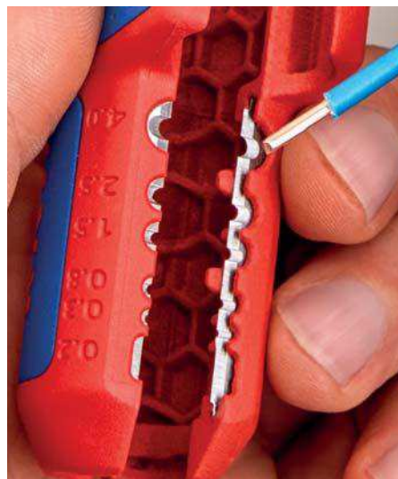
Abisolieren von Einzelleitern
